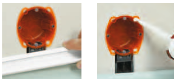
Проверка правильности расположения коробки и мини-каналов
